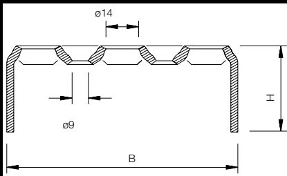
Planke 14/9 – tværsnit
