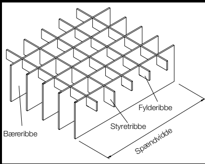
Skærerist
