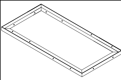
V-stålrammer med boltehuller i vandret eller lodret flance
